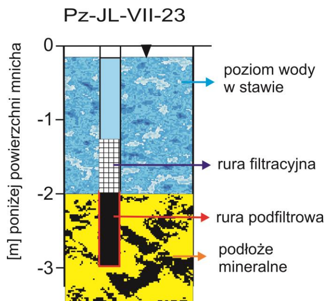
Rycina 23. Limnimetr/piezometr nr Pz_IL-VII-23 – Imielty Ług VII
