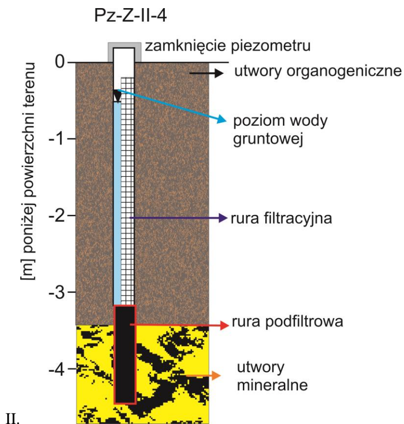
Rycina 4. Piezometr nr Pz_Z-II-4 – Zdzisławice II
