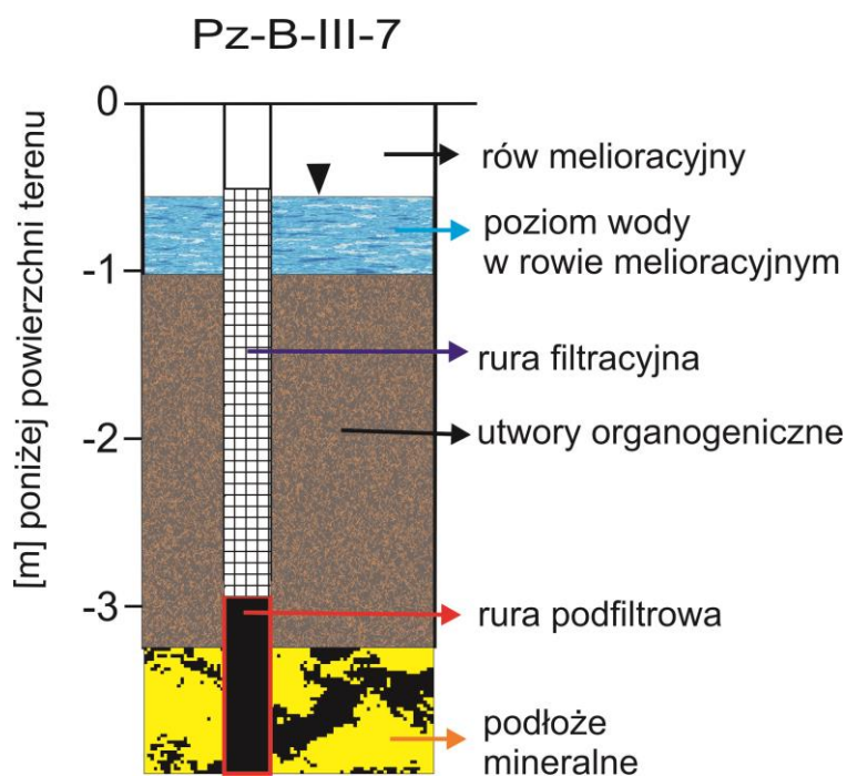
Rycina 7. Limmimetr/piezometr nr Pz_B-III-7 – Bukowa III
