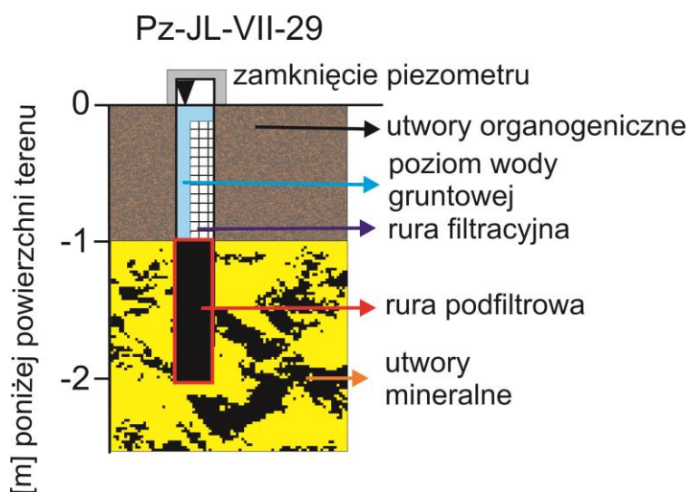
Rycina 29. Piezometr nr Pz_IL-VII-29 – Imielty Ług VII
