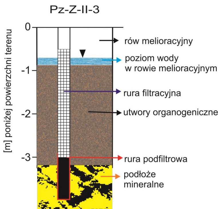
Rycina 3. Limmimetr/piezometr nr Pz_Z-II-3 – Zdzisławice II
